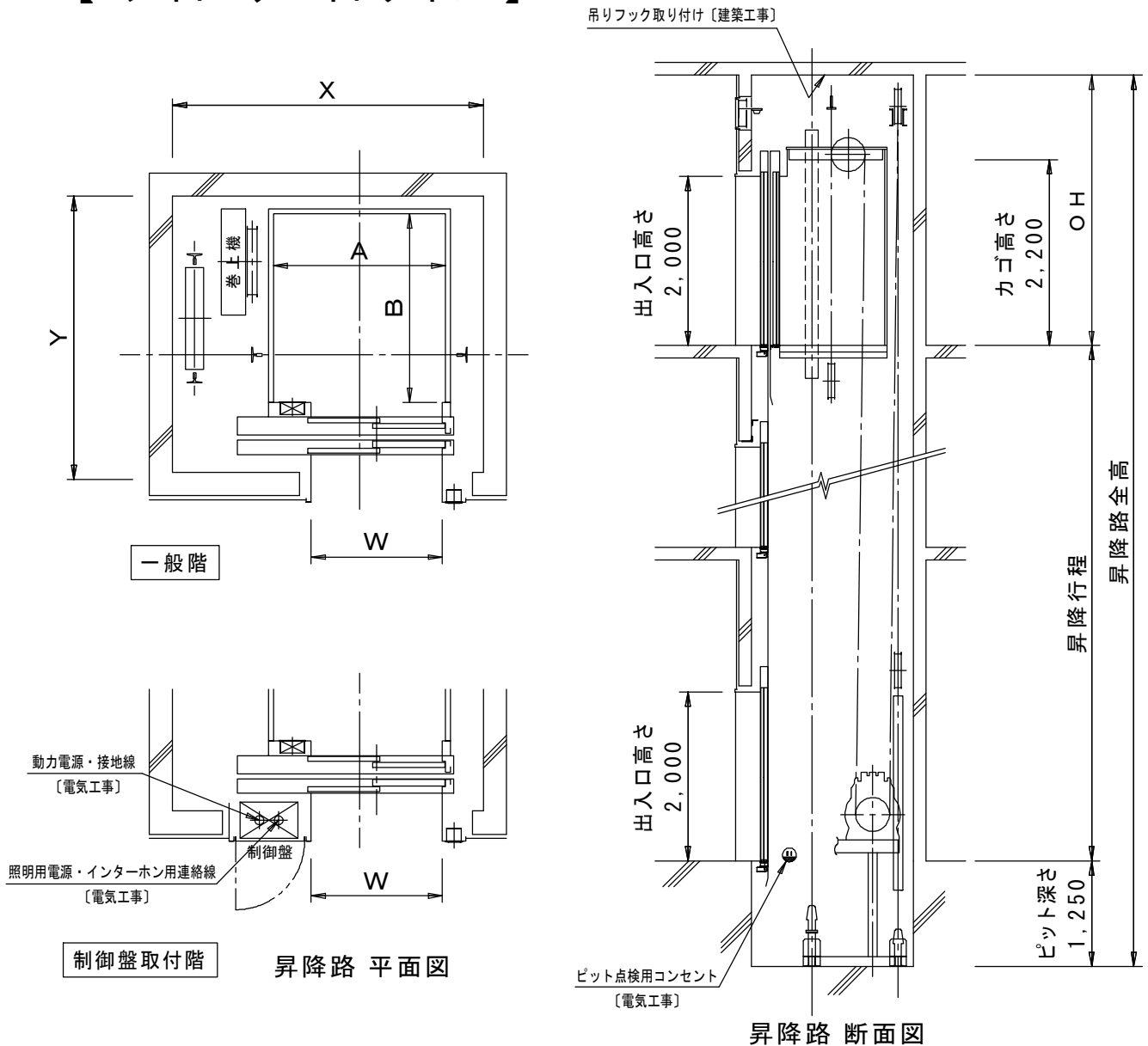
住宅用エレベーター 寸法一覧表
